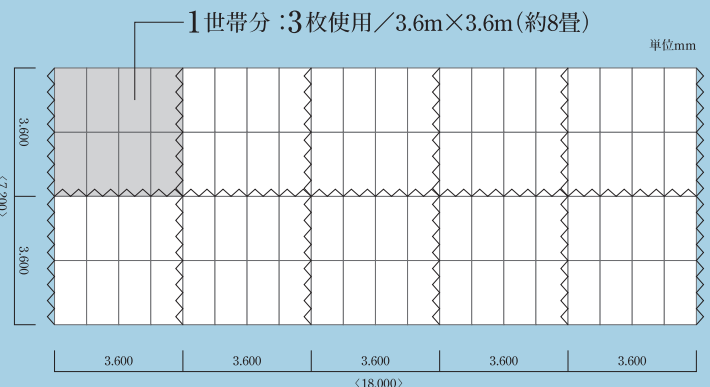
【10世帯分配置図】 17枚使用
